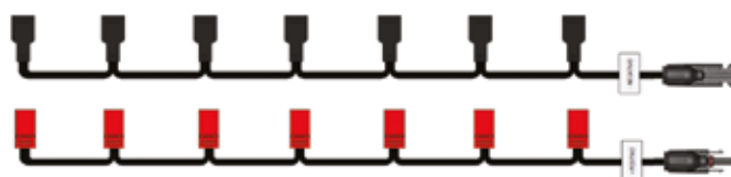
Cabeamento para o Paralelo de 7 séries
